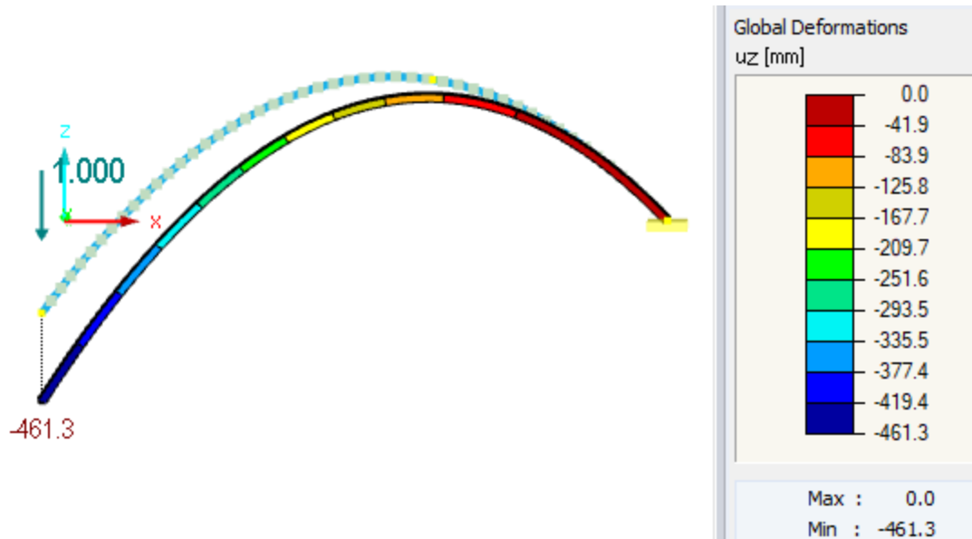
Figura 7 Deformación vertical por carga unitaria vertical
