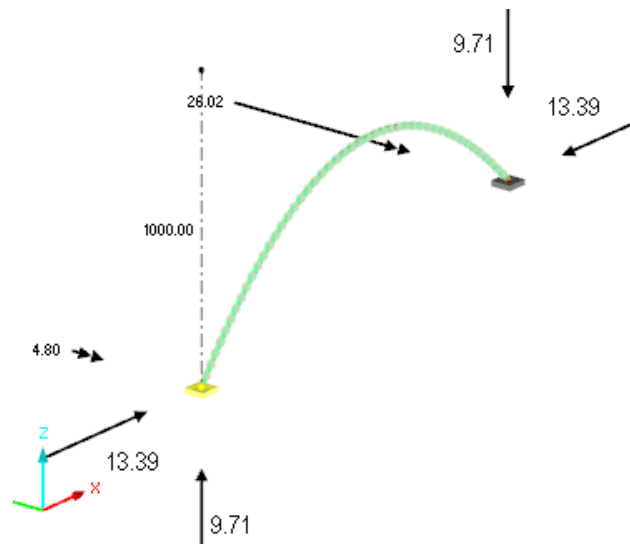
Figura 30 Reacciones en apoyos de arco parabólico
