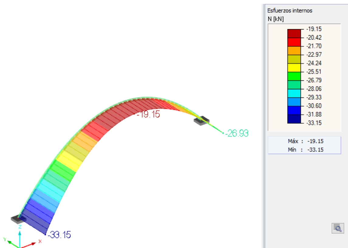
Figura 33 Diagrama de cargas axiales
