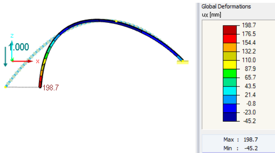
Figura 8 Deformación horizontal por carga unitaria vertical
