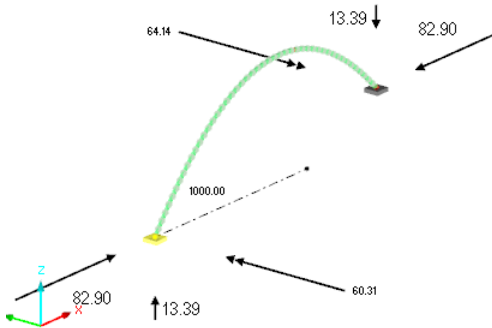
Figura 31 Reacciones en apoyos de arco parabólico
