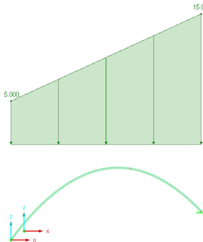
Figura 22 Carga trapezoidal externa proyectada sobre viga en forma de arco parabólico.
