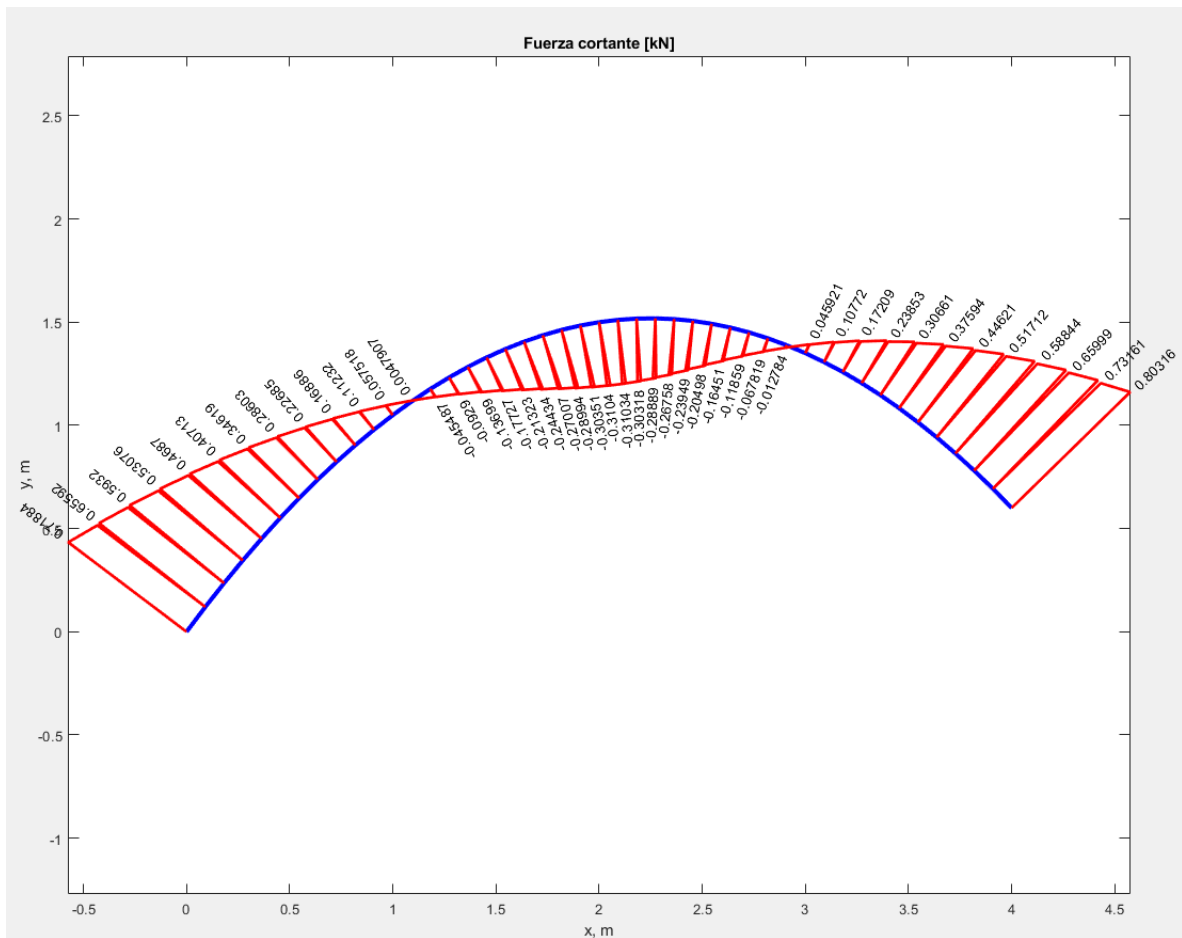
Figura 36 Diagrama de fuerzas cortantes
