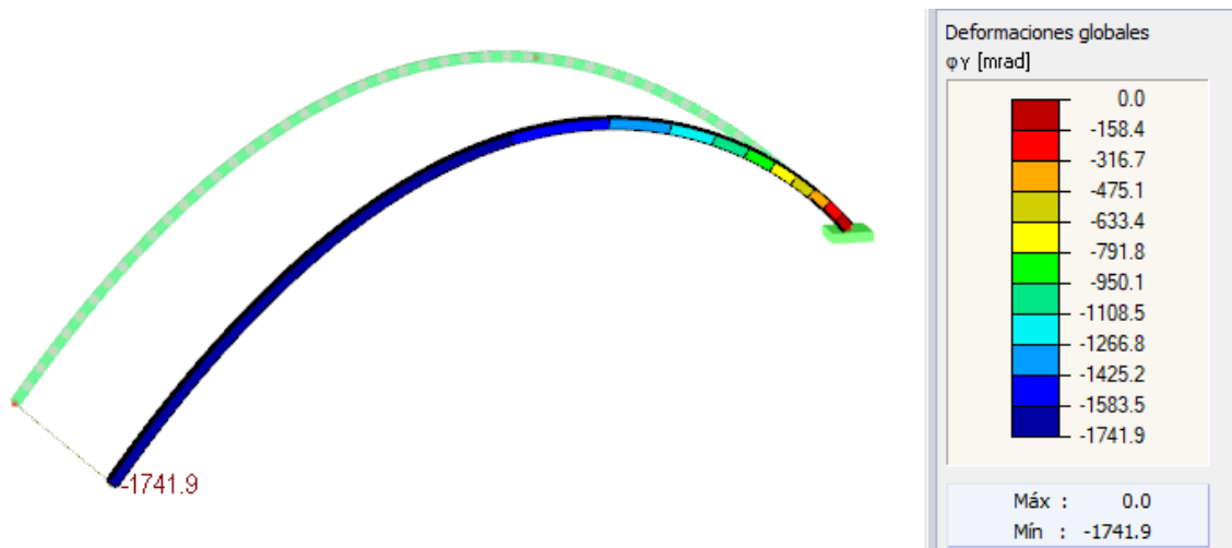
Figura 28 Ángulo de giro por carga trapezoidal vertical
