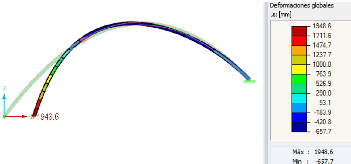
Figura 27 Deformación horizontal por carga trapezoidal vertical
